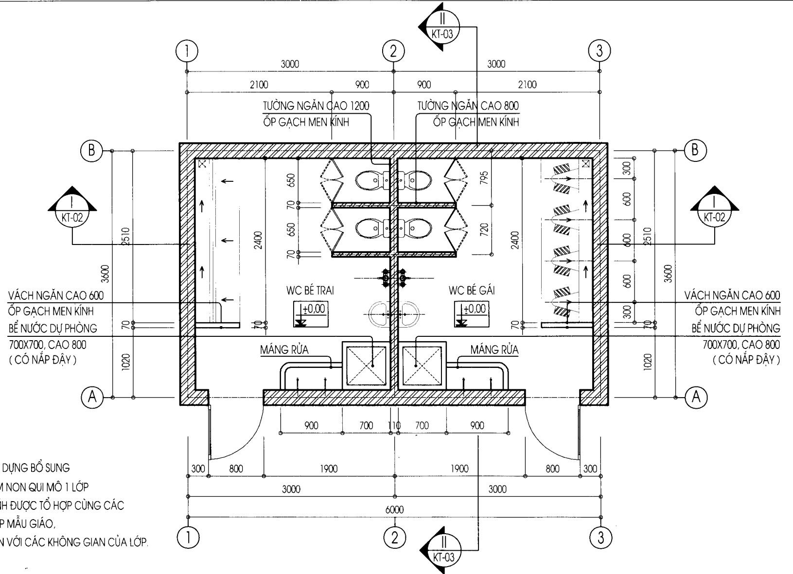
MẶT BẰNG KHU VỆ SINH
